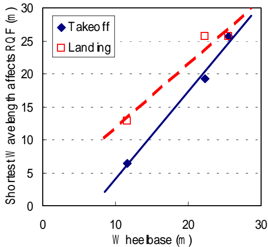
図-12 航空機のホイールベースとRQFに影響する最短波長の関係
