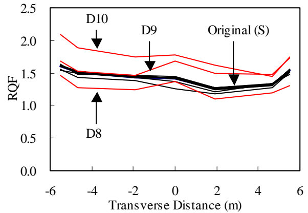
図-7 横断位置とRQFの関係 (B-747, R34, 着陸)
