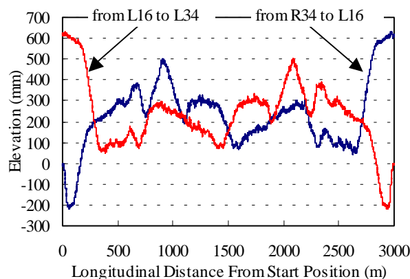
図-3 測定したプロファイルの例 (Line4)
