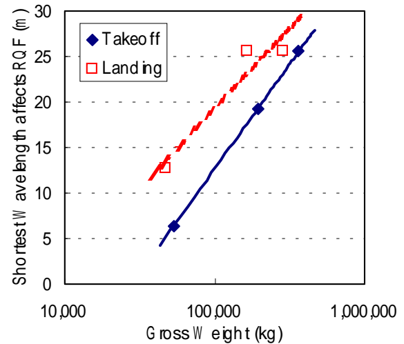
図-13 航空機の総重量とRQFに影響する最短波長の関係
