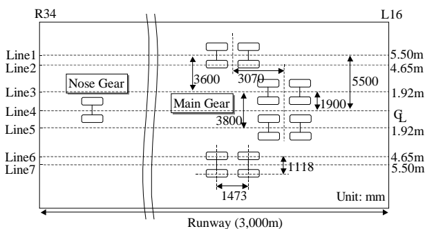
図-2 プロファイルの測線とB747のギア構成
