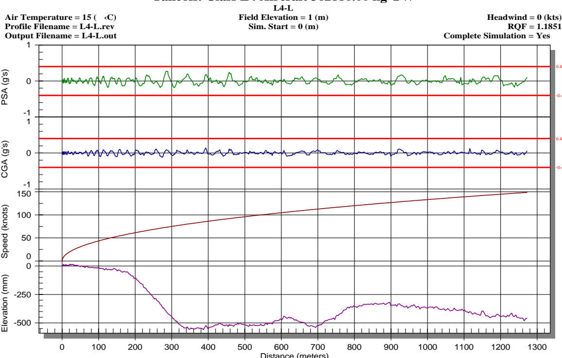
図-4 APRas による航空機の鉛直加速度のシミュレーション結果 (Line4, 離陸の例)
