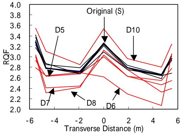
図-9 横断位置とRQFの関係 (B-737, R34, 離陸)
