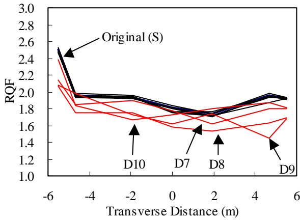
図-6 横断位置とRQFの関係 (B-747, R34, 離陸)
