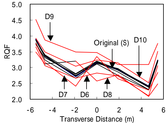
図-11 横断位置とRQFの関係 (B-737, R34, 着陸)
