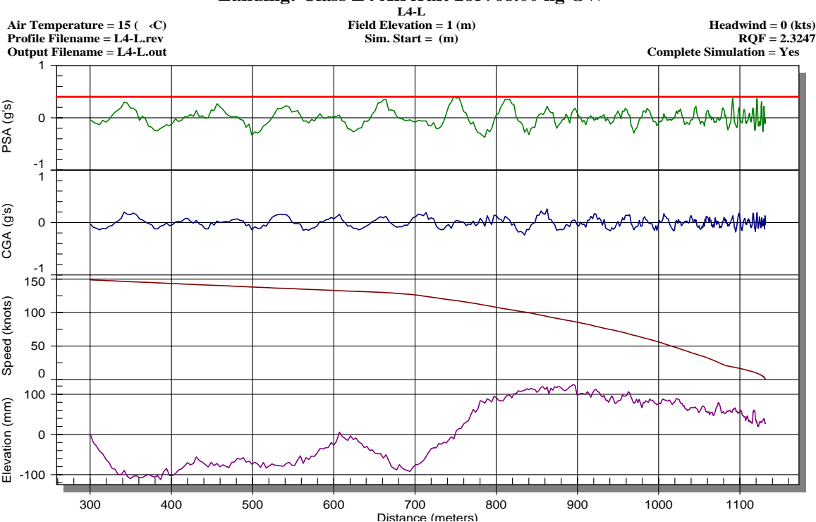
図-5 APRas による航空機の鉛直加速度のシミュレーション結果 (Line4, 着陸の例)
