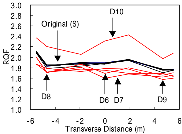
図-8 横断位置とRQFの関係 (DC-10, R34, 離陸)
