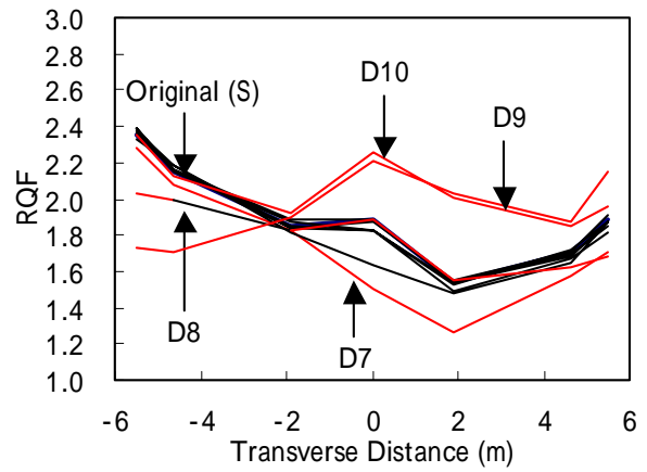
図-10 横断位置とRQFの関係 (DC-10, R34, 着陸)
