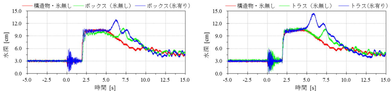
図-3 PG3 (x=2.83 m)地点で計測された時系列的な水深の変化 (左段がボックス, 右段がトラス橋の場合)
