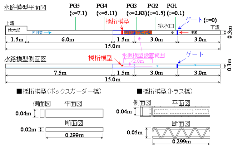
図-1 使用した水路及び橋梁模型の平面図・側面図
