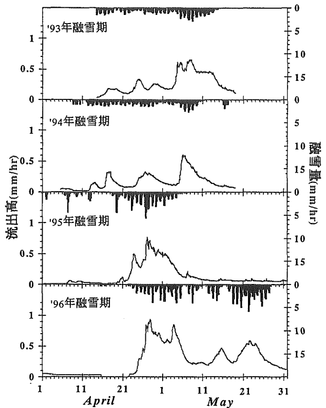
図-2 1993～1996年融雪期の流量ハイドログラフ
