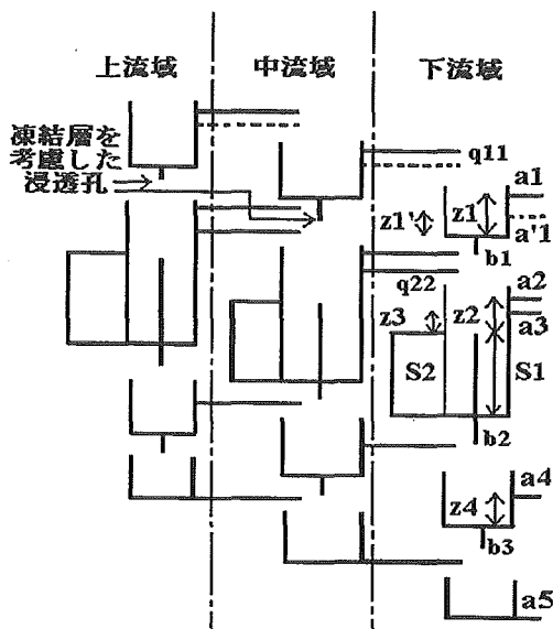
図-5 三列四段タンクモデル
