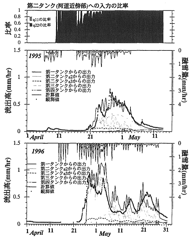
図-8 '95,'96年融雪期再現計算結果
