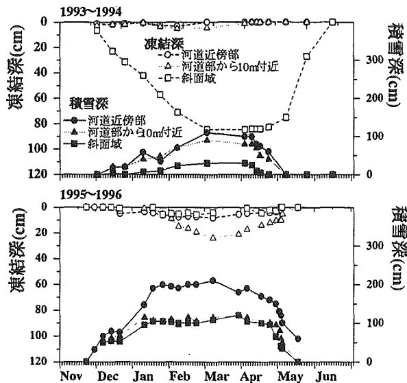
図-3 1994,1996年の凍結深・積雪深変化
