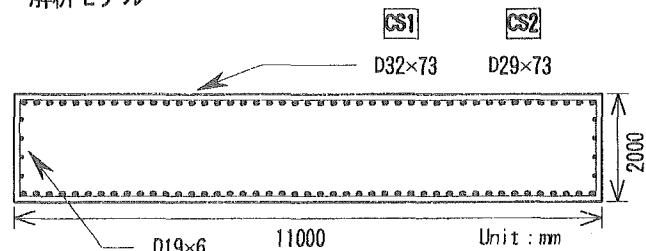
図-2 橋脚断面
