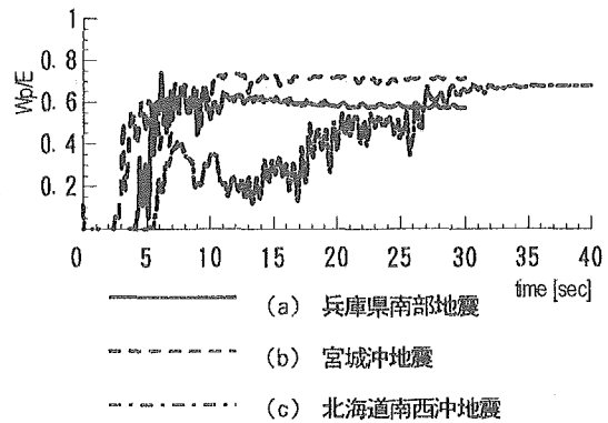
図-5 応答変位
