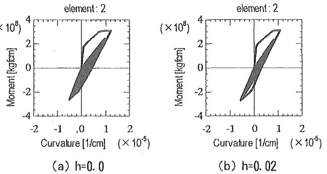
図-8 M- \phi 曲線
