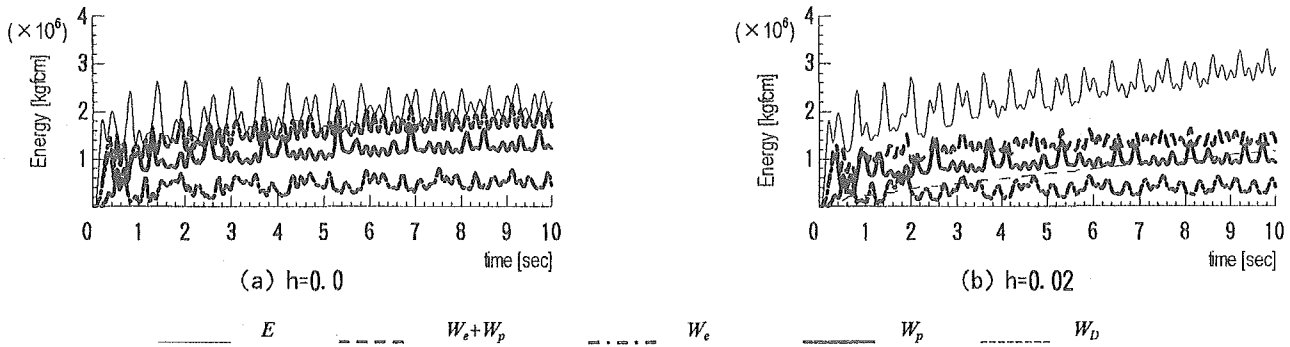
図-7 エネルギー収支
