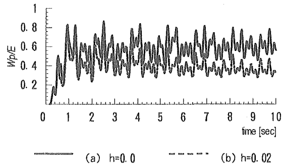
図-9 W_p/E 時刻歴
