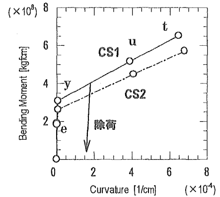
図-3 M-φ曲線モデル
