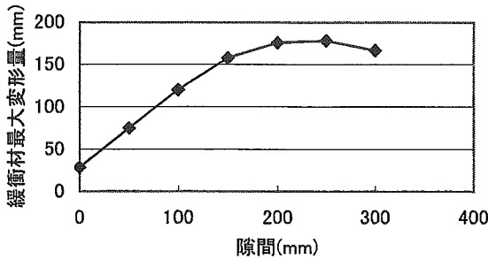
図-12 緩衝材の最大変形量の変化
