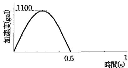
図-5 入力加速度
