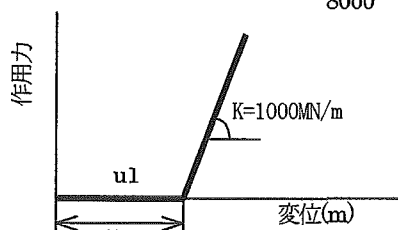
図-4 衝突バネモデル
