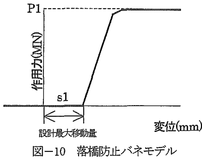
図-10 落橋防止バネモデル
