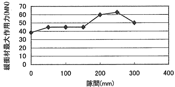
図-13 緩衝材の最大作用力の変化
