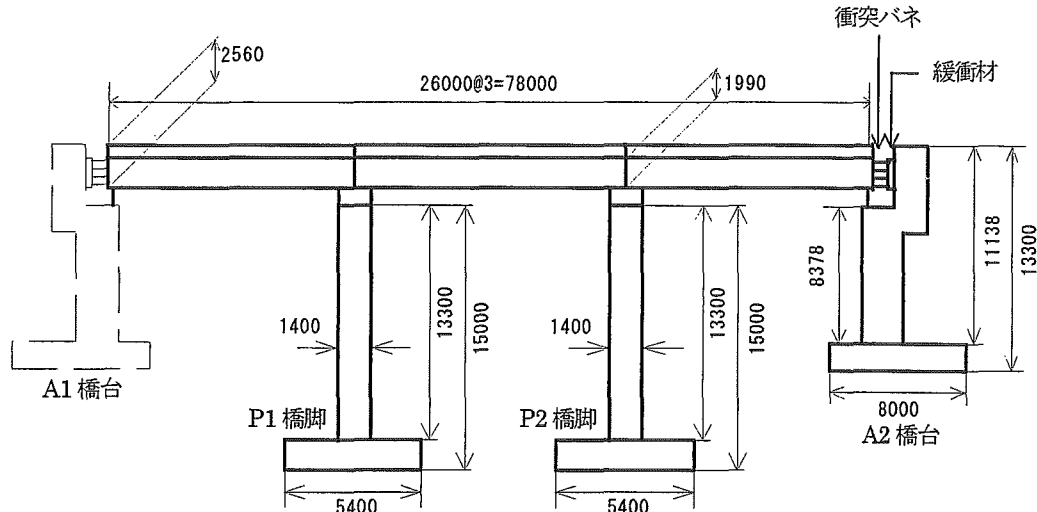
図-11 連続桁橋解析モデル図
