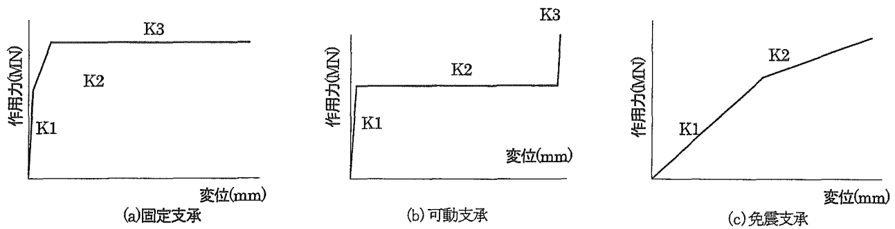
図-6 支承モデル
