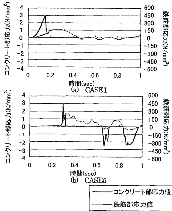
図-15 橋台基部の曲げ応力値の比較
