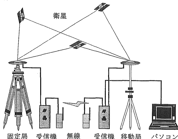
図一2 測定イメージ
