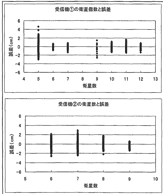
図-8 各受信機の衛星数と誤差
