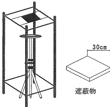
図-3 遮蔽物による衛星状態測定
