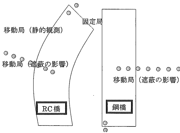
図-4 橋梁下における移動局（静的観測）衛星状態測定と桁端上部モニタ固定局
