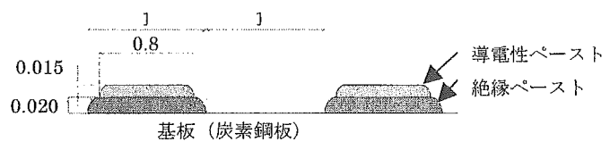
図-2 ACM センサ断面図 (単位: mm)
