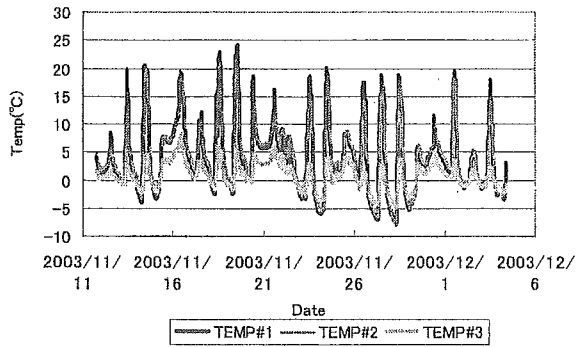
図-5 温度センサ出力状況
