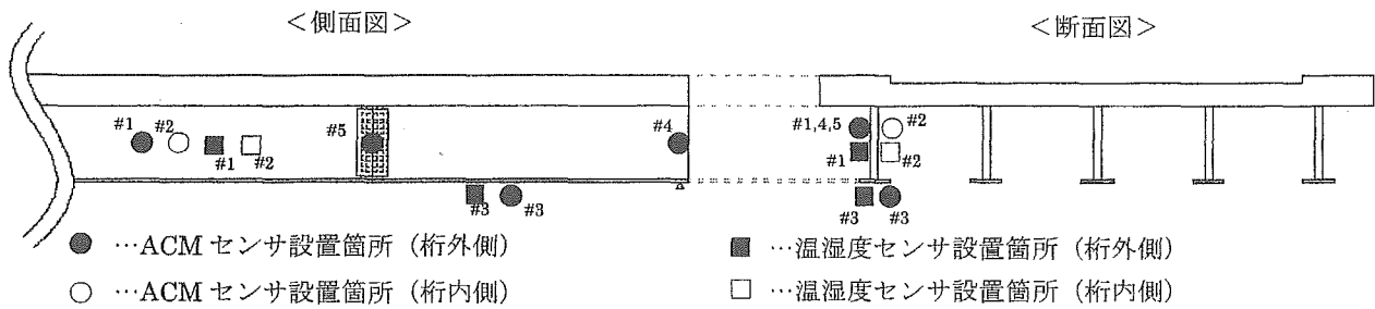
図-3 ACM センサおよび温湿度計設置箇所
