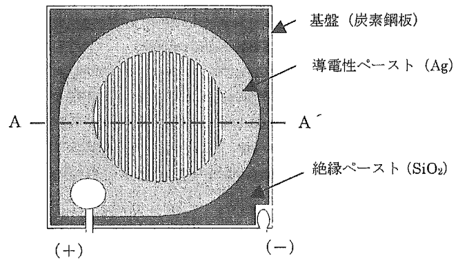
図-1 ACM センサ平面図
