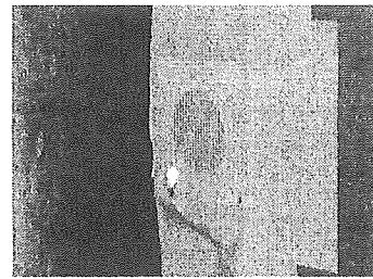
写真-1 桁端部 ACM センサ取り付け状況
